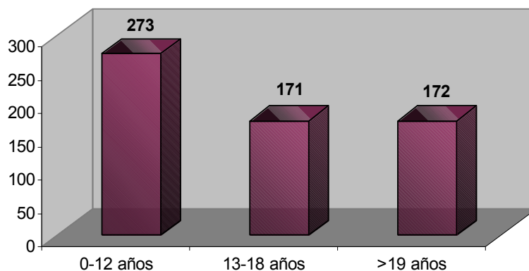
Fig. 3. Número de artículos según rango de edad estudiada
