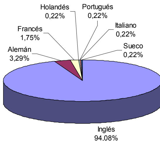
Fig. 4. Número de artículos según idioma
