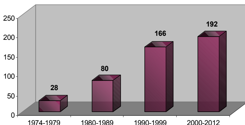
Fig. 1. Número de artículos publicados por años
