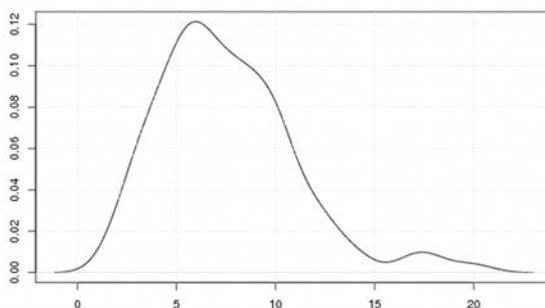
Figural: Análisis de densidad de Kernel para función Gaussiana. Eje Y: Densidad para cada valor de Folato sérico; Eje X: Folato sérico
