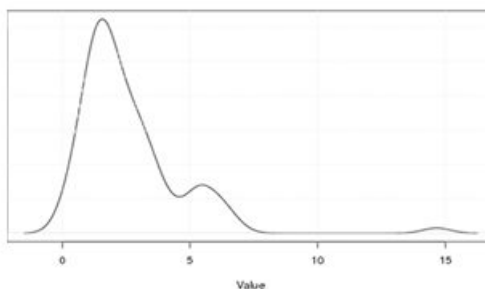
Figura 3 Análisis de densidad de Kernel para función Gaussiana. Eje Y: Densidad para cada valor de TSH, Eje X: TSH
